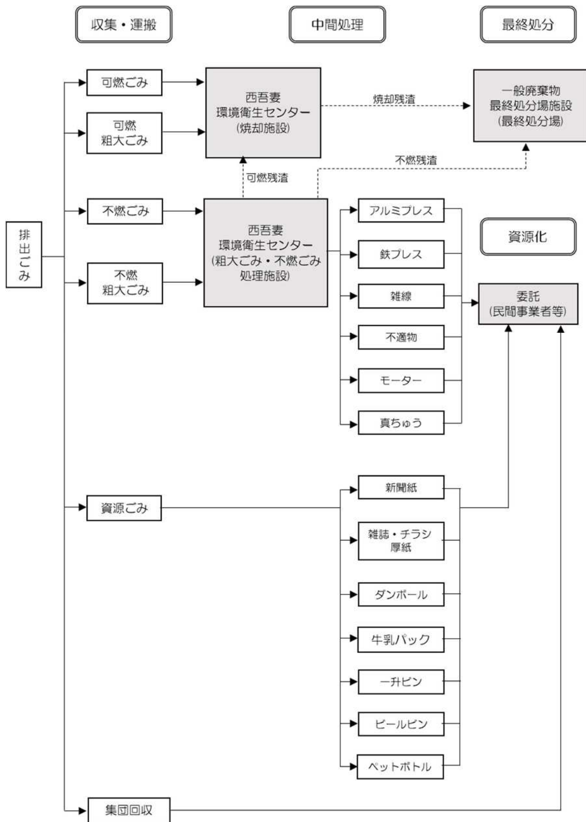
図 2-1-1 (2) ごみ処理・処分の流れ (西吾妻環境衛生施設組合)
